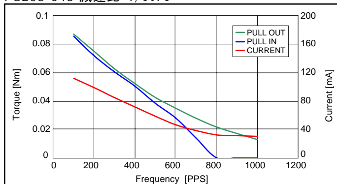
PG25S-048 減速比 1/236
