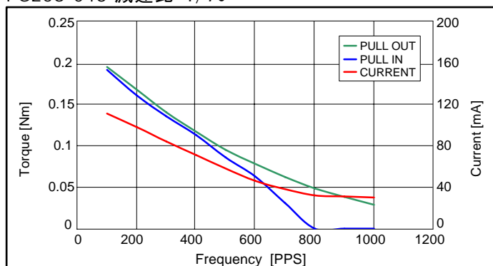
PG25S-048 減速比 1/76
