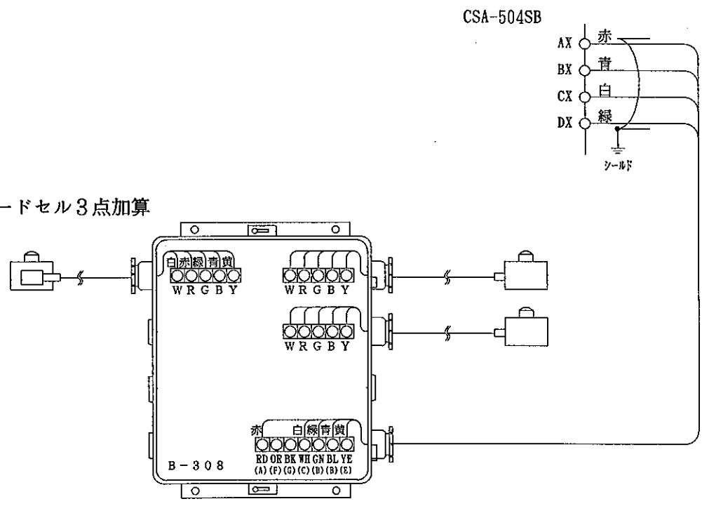
加算型ジャンクションボックス
