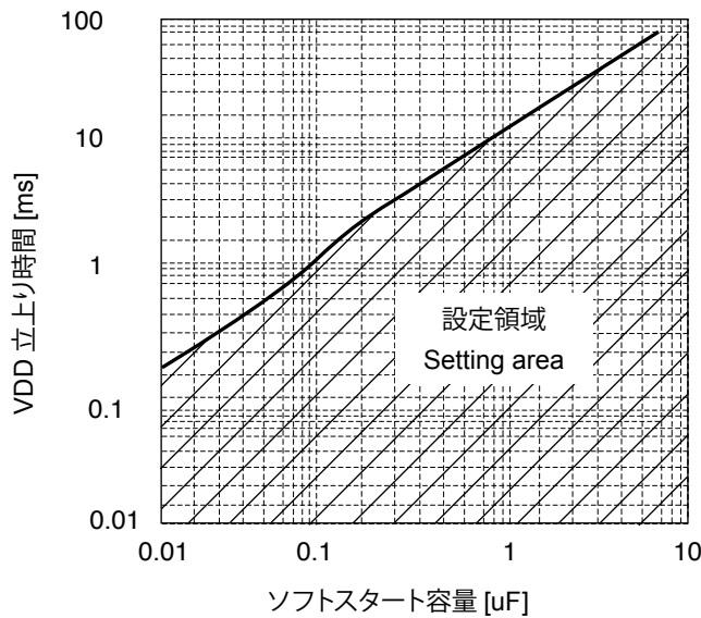
Fig.1 ソフトスタート容量 vs VDD 立ち上がり時間
